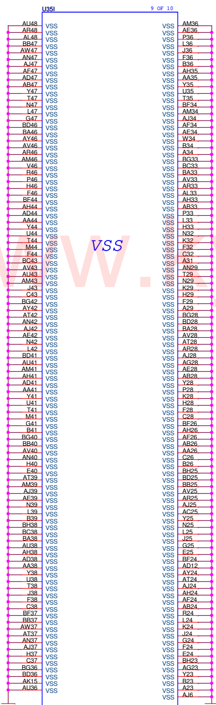
CANTIGA-GM-GP-U-NF 71.CNTIG.00U
