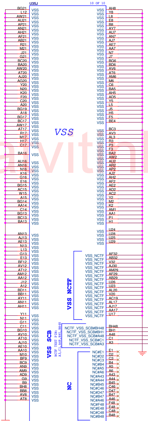
CANTIGA-GM-GP-U-NF 71.CNTIG.00U
